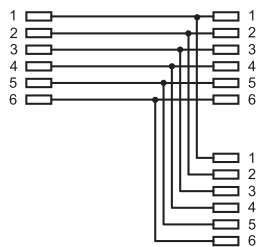
Schaltbild Wiring diagram
