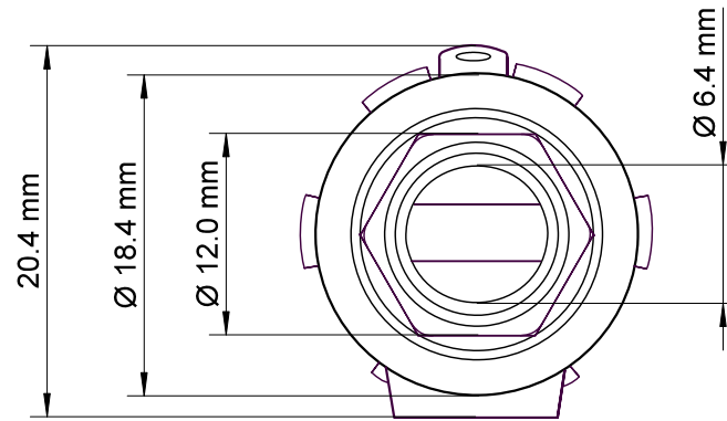
Unterlegscheibe washer
