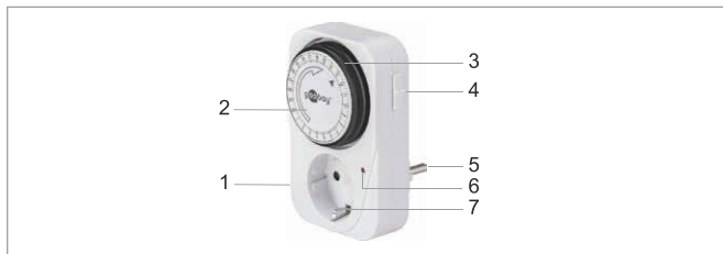
Fig.41: Tuotteen osat
